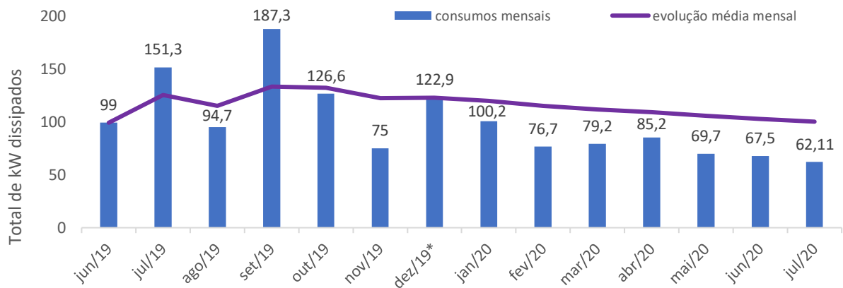
Figura 3 - Evolução da potência elétrica dissipada em kW:
